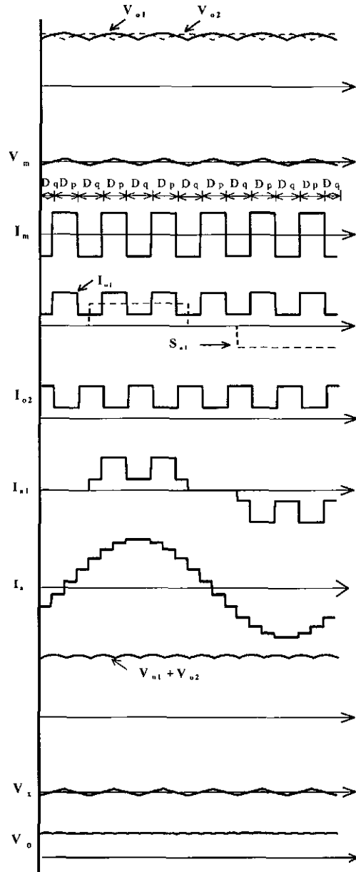
그림 2 계산 결과 ( K=0.984 , I_o=1(PU) , V_{LL}=1(PU) 일 때) Fig 2 Calculation results (Assuming k=0.984 , I_o=1(PU) and V_{LL}=1(PU) )
