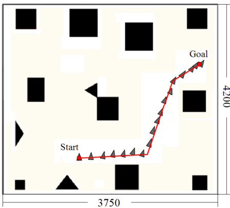
그림 17. 이동로봇 추종제어 실험결과.
