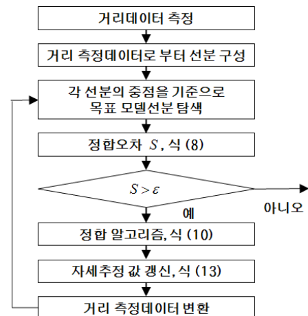
그림 12. 정합 알고리즘 흐름도. Fig. 12. Matching algorithm flow chart.
