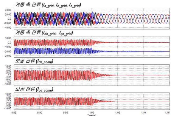
그림 14 능동댐핑 적용 전후의 전류 파형 Fig. 14 Simulated current waveform without and with active damping method
