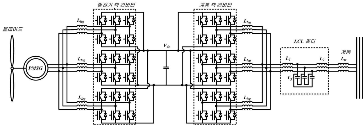
그림 1 3병렬 풍력발전 시스템 구성
