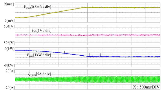
그림 24 MPPT 운전시 실험 결과
