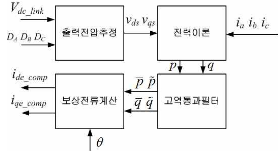
그림 7 전력이론을 이용한 보상기 블럭도
