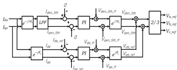
그림 10 5차 고조파 제어가 추가된 전류 제어 루프
