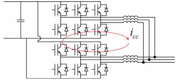
그림 3 병렬 운전에 의한 순환전류
