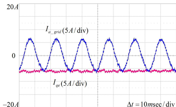
그림 22 출력전류와 q축 전류 (불평형 및 왜곡 보상 후)
