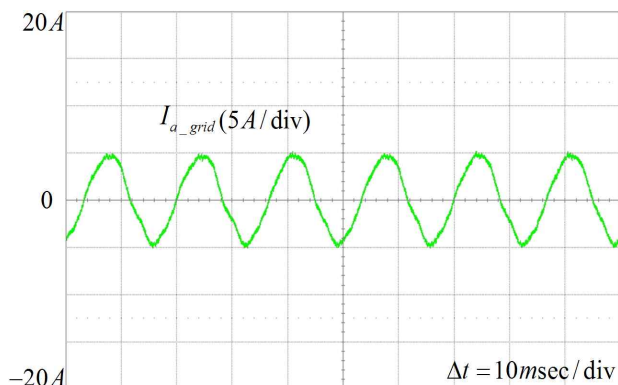
(b) 능동댐핑 적용 후
