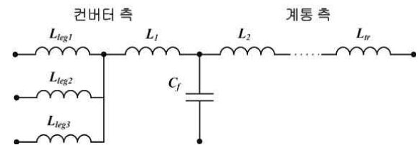
그림 4 계통 측 LCL 필터의 단상 등가 회로
