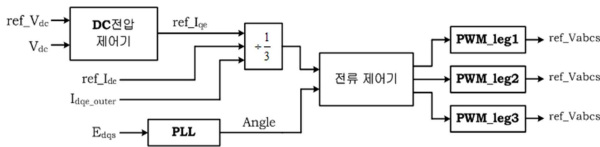
그림 2 외부 제어 블록도
