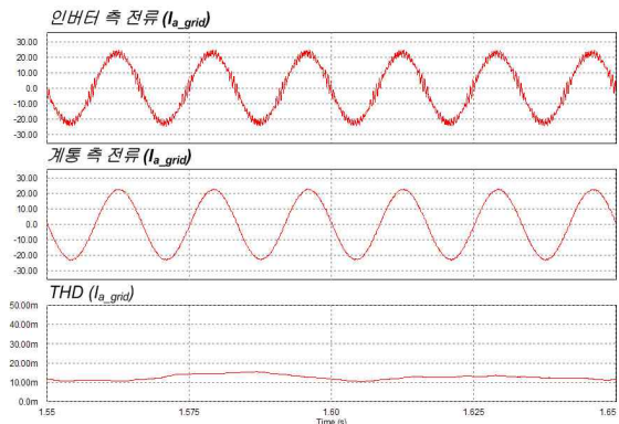
그림 13 LCL필터의 성능 Fig. 13 The performance of the designed LCL filter
