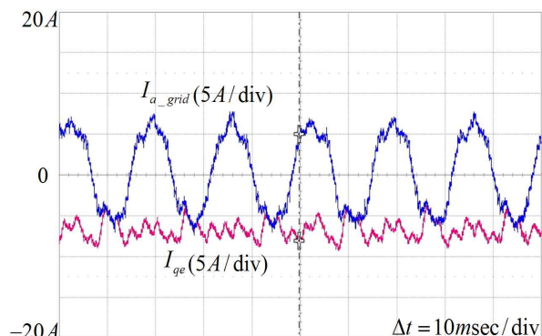
그림 20 출력전류와 q축 전류 (보상 전)
