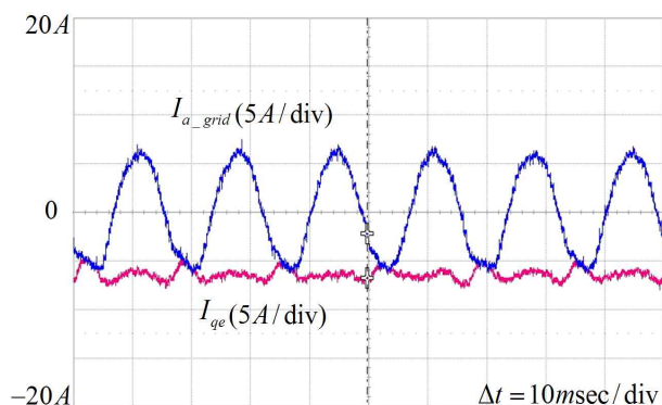
그림 21 출력전류와 q축 전류 (왜곡 보상 후)
