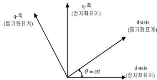
그림 6 고정좌표계에서 동기좌표계로의 변환
