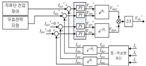
그림 8 계통 전압 불평형시 보상 제어 블록도 Fig. 8 The control scheme with compensation of the grid voltage unbalance.
