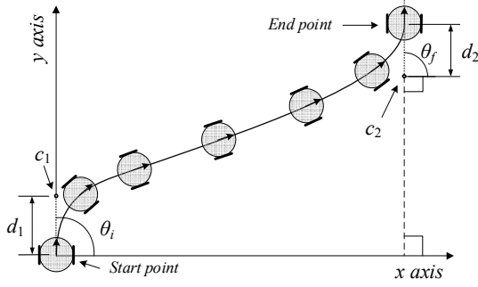
그림 1. 베지어 곡선 기반 S-곡선 경로.
