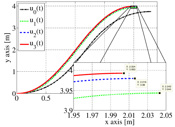
그림 4. 에러 보정 u(t) 에 의해 생성된 경로계획.
