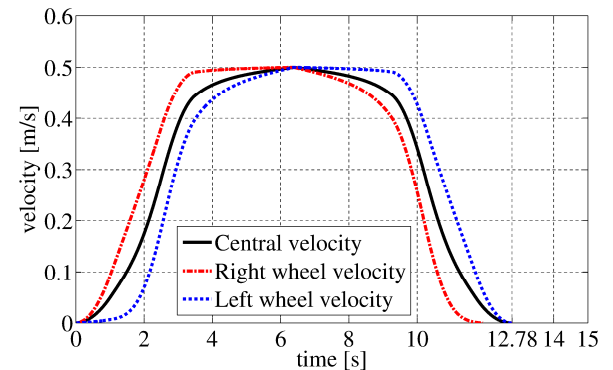
그림 7. 두 바퀴의 물리적 제한을 고려한 속도 명령.
