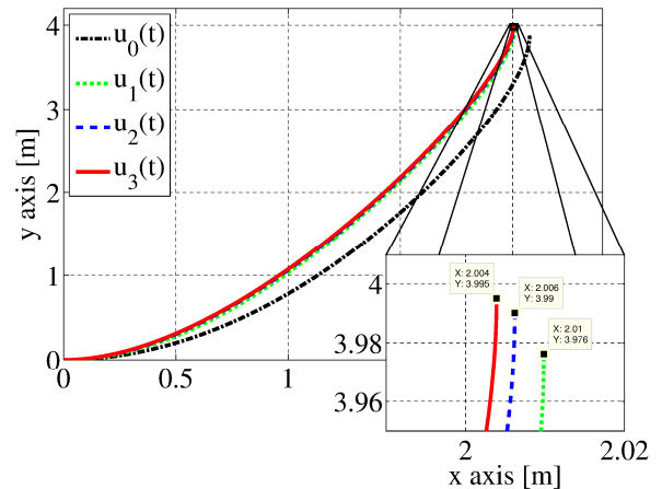
그림 10. 수치적으로 계산된 경로계획 (C-curve path).
