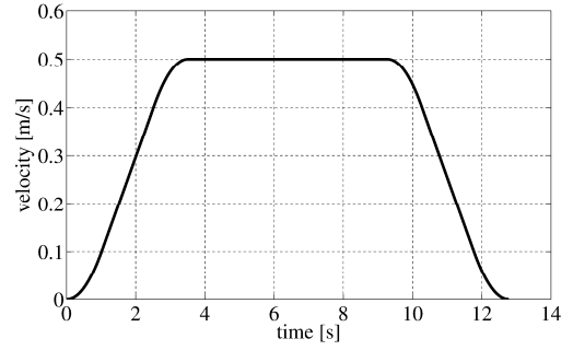
그림 2. 컨볼루션 연산 기반 이동로봇의 중심 속도궤적.
