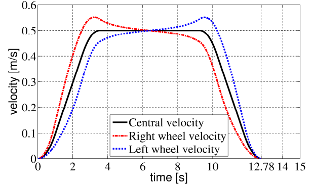
그림 6. 두 바퀴 이동로봇의 속도 명령.
