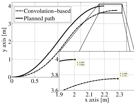
그림 3. 이동로봇 중심의 물리적 제한이 고려된 경로계획.
