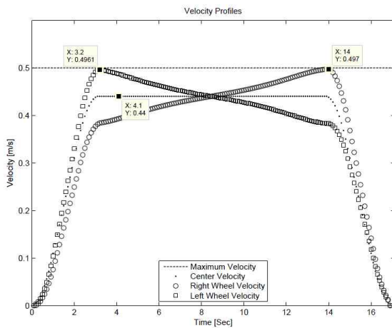
그림 5. 시스템 제한이 고려된 관절 속도 명령.
