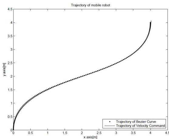
그림 6. 직교좌표계에서 TMR의 궤적.
