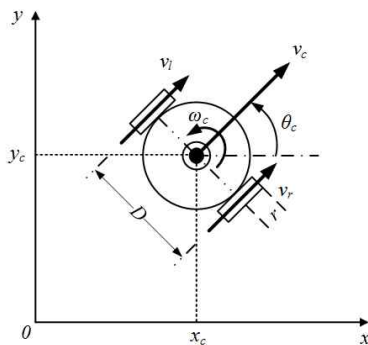
그림 3. TMR의 기준 좌표계.
