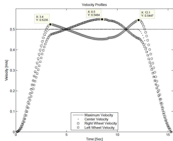
그림 8. 콘볼루션을 통하여 구한 관절 속도 명령.
