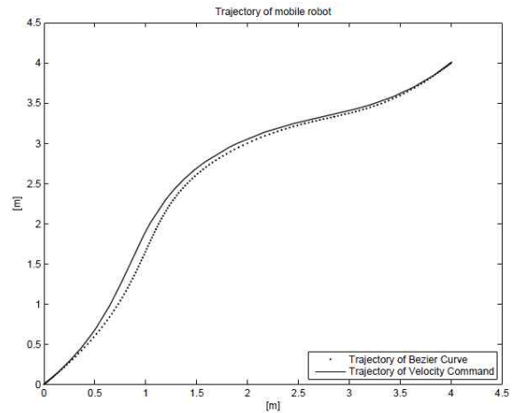
그림 11. 연속적인 경로에서 TMR의 궤적.
