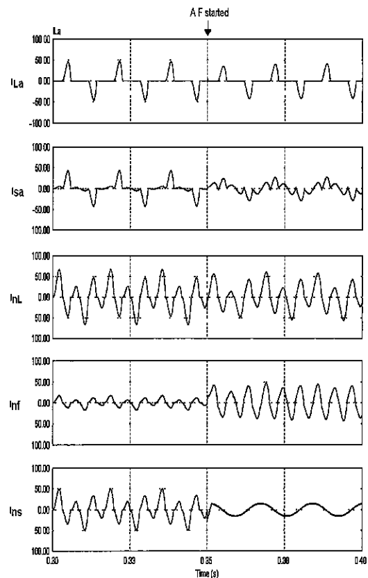
그림 5 부하불평형(UBF=30%)일 때 시물레이션 파형
