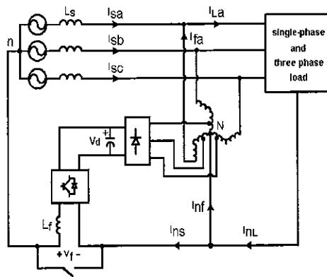
그림 1 제안한 능동전력필터 시스템 Fig 1 Proposed active power filter system
