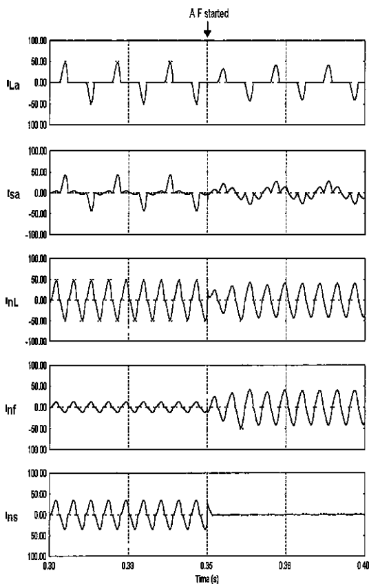
그림 4 부하평형일 때 시물레이션 파형
