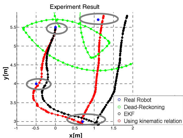
그림 13. 실시간 위치추정 실험 결과. 추측항법(연두색), EKF (검은색), 기구학적 관계를 이용한 EKF(빨간색).
