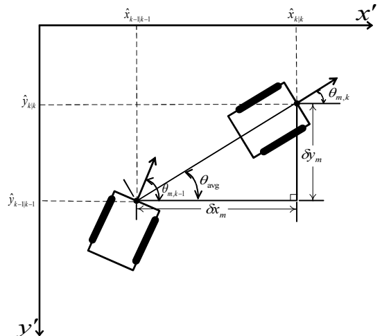
그림 4. 기구학적 관계를 이용한 보정모델 도출.
