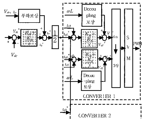
그림 3 PI 제어기에 의한 병렬운전 PWM 컨버터의 제어선도
