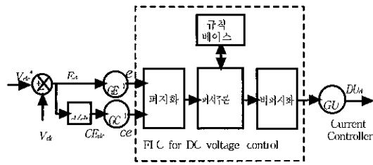
그림 5 직류전압 제어를 위한 퍼지 제어기의 블록도 Fig. 5 Block diagram of FLC for DC voltage control
