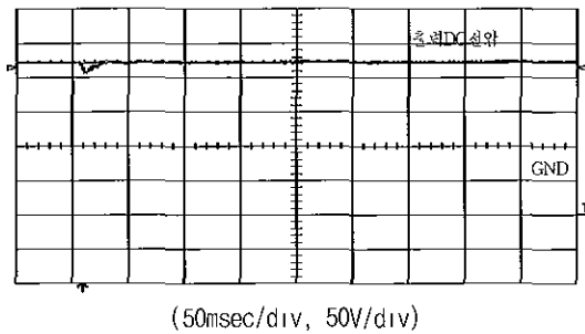
그림 23 출력 직류전압의 과도 응답 특성 Fig 23 Transient response characteristic of DC output voltage
