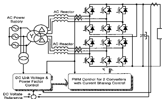
그림 1 병렬운전 PWM 컨버터의 구성도
