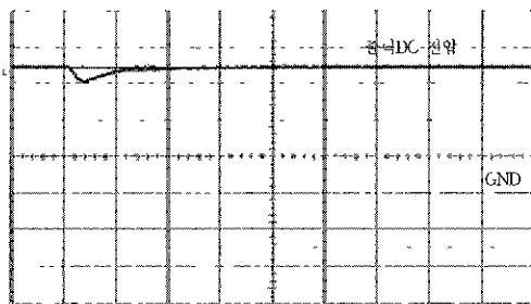
그림 20 출력 직류전압의 과도 응답 특성
