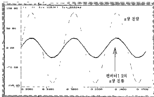
그림 11 역률 제어 파형 특성 Fig 11 Waveform characteristics of power factor control
