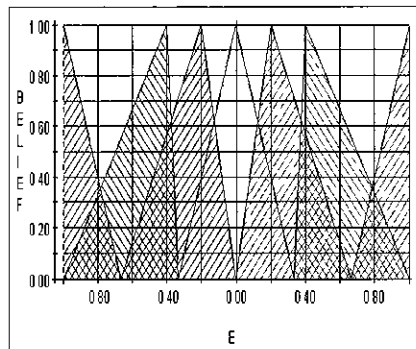
그림 6 오차( E_{dc} )의 소속함수 Fig. 6 Membership functions of error( E_{dc} )
