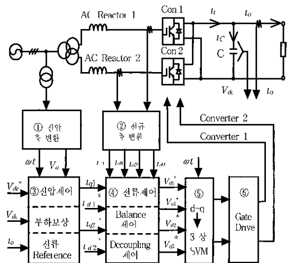
그림 2 병렬운전 PWM 컨버터의 제어 블록도
