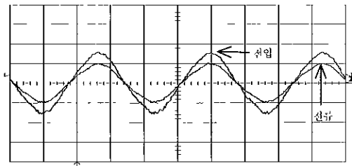
그림 19 역률 제어 파형 특성
