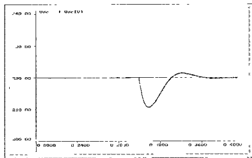
그림 12 스텝 부하 인가시 직류전압 응답 특성 Fig 12 DC voltage response characteristics to step increase of load
