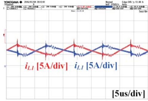
(d) i_{L1} , i_{L2}
