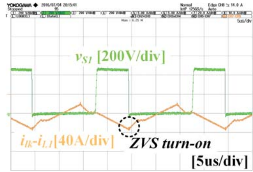
(e) i_{S1} , v_{S1}
