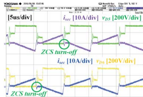
(g) i_{D5} , i_{D6} , v_{D5} and v_{D6}
