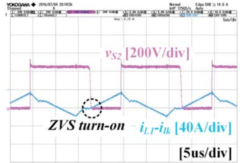
(f) i_{S2} , v_{S2}
