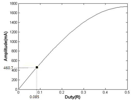
(a) 튜티비에 따른 부하전류의 진폭
