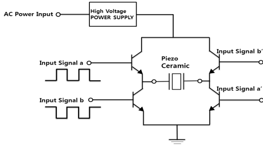
(b) H-브리지 앰프 방식
