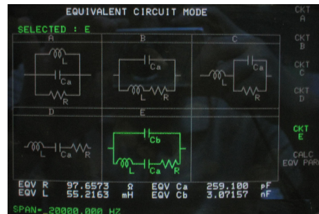
(b) 등가 회로 모델
