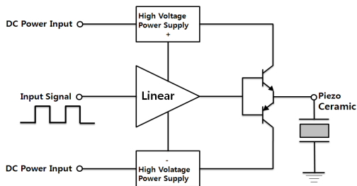
(a) 선형앰프 방식
