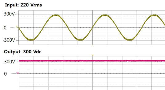
[그림 11] 전원장치 입출력 전압 파형 [Fig. 11] Input-output voltage waveform of power supply
