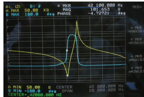
(a) 주파수에 따른 임피던스 응답
