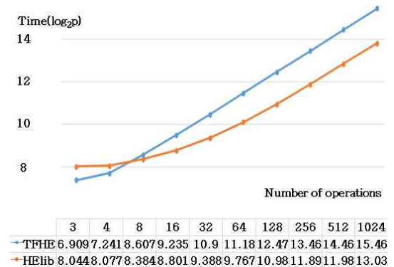
그림 8. HELlib, TFHE에서 64bit 덧셈 연산 시간 비교 Fig. 8. Comparison of execution time for 64bit addition in HELlib, TFHE
