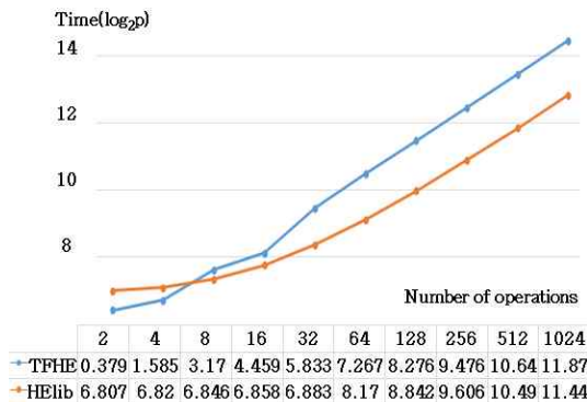
그림 6. HELib, TFHE에서 32bit 덧셈 연산 시간 비교 Fig. 6. Comparison of execution time for 32bit addition in HELlib, TFHE
