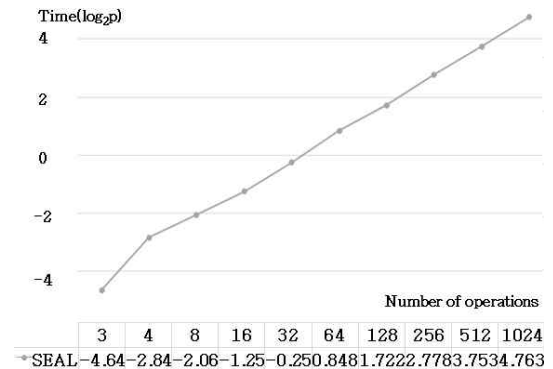
그림 9. SEAL에서 64bit 덧셈 연산 시간 비교 Fig. 9. Comparison of execution time for 64bit addition in SEAL
