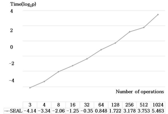
그림 7. SEAL에서 32bit 덧셈 연산 시간 비교 Fig. 7. Comparison of execution time for 32bit addition in SEAL
