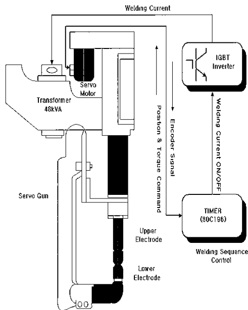
그림 2 서보건을 이용한 저항 스폿용접 시스템
