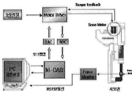
그림 11 선형특성 실험을 위한 시스템 구성 Fig. 11 System configuration for linear characteristics test
