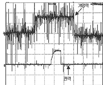
(b) 가압력 명령치:400[kgf], 정전력 명령치:7[kW] 일 때
