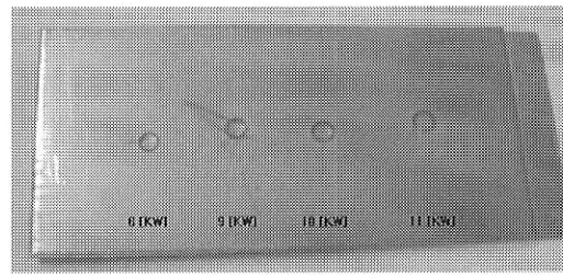
(a) 정전력 : 8-11 [kW], 가압력 : 200 [kgf], 용접시간 : 120 [ms]
