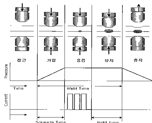
그림 1 용접 공정별 전극의 제어
