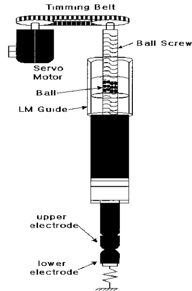
그림 3 서보건의 내부구조
