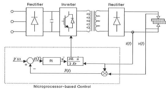
그림 9 선형화 제어를 위한 블록선도 Fig. 9 Block diagram for linearized control
