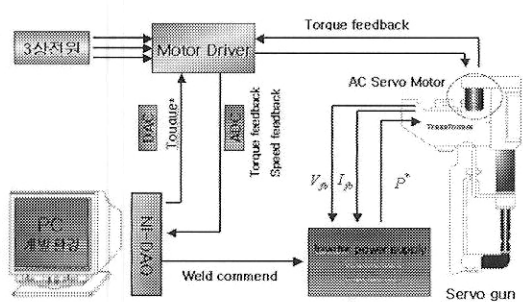
그림 13 용접품질시험 구성도
