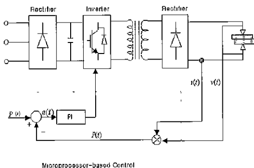
그림 5 정전력 제어 시스템의 블록선도 Fig 5 Block diagram of constant power control system
