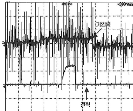
(a) 가압력 명령치:180[kgf], 정전력 명령치:7[kW] 일 때
