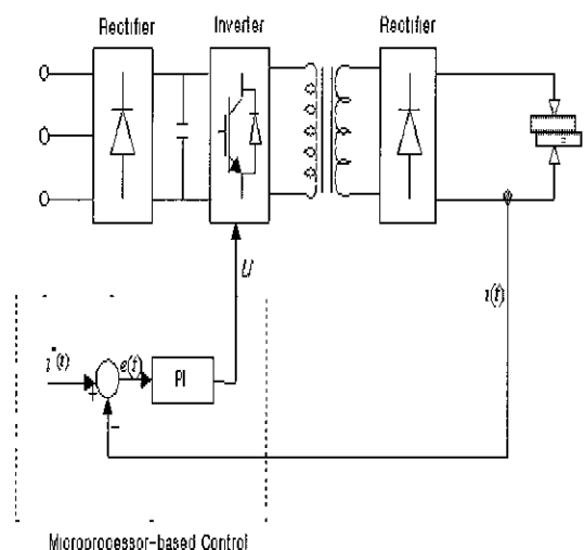
그림 4 정전류 제어시스템의 블록선도
