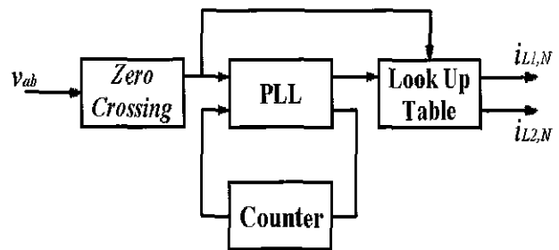
그림 5 지령전류 발생
