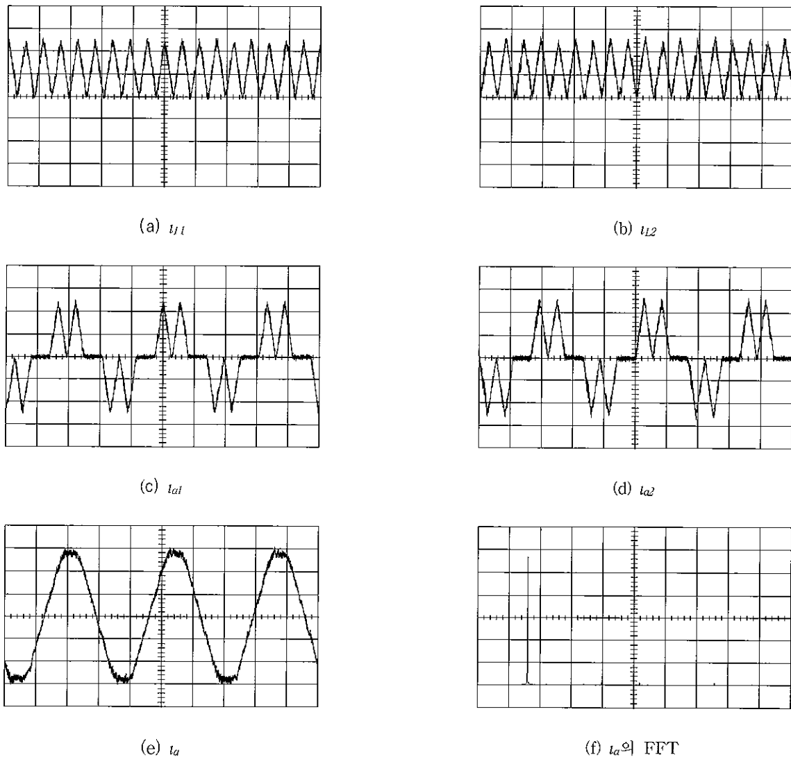
그림 8 실험파형(Waveforms 2A/div, 5ms/div, FFT 1A/div, 100Hz/div) Fig 8 Experimental waveforms(Waveforms 2A/div, 5ms/div, FFT 1A/div, 100Hz/div)
