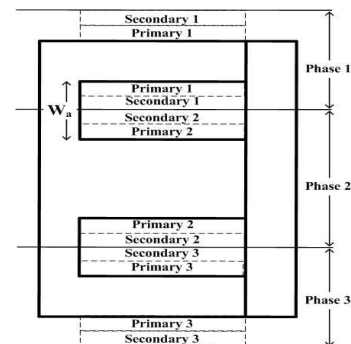
그림 5 EI코아의 3상 권선 방법
