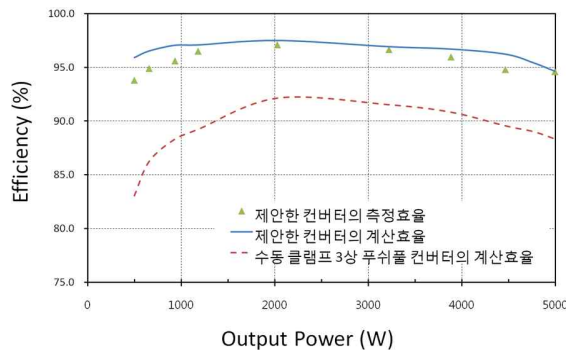
그림 17 측정된 효율
