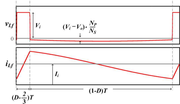
그림 11 입력필터 인덕터의 전압과 전류 파형
