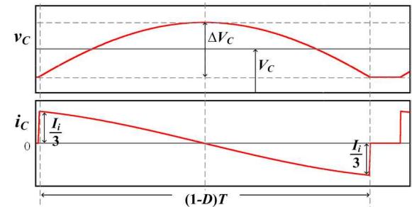
그림 12 클램프 커패시터의 전압과 전류 파형
