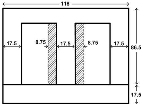
그림 8 커팅후 티코아 (단위:mm)
