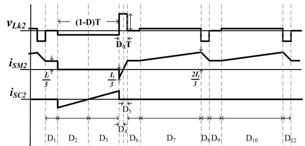
그림 4 메인스위치와 클램프스위치 전류파형
