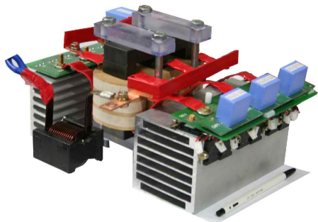
그림 14 5kW급 시작품 사진
