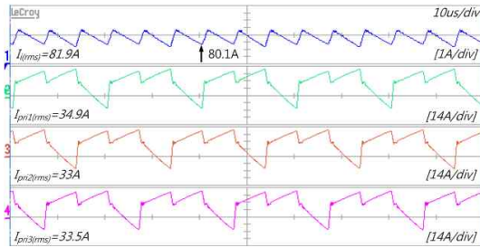
(c) 권선 전류 파형
