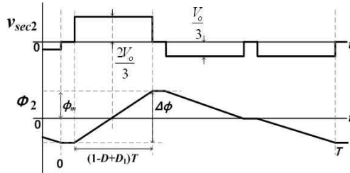
그림 6 변압기 2차측 전압과 자속파형
