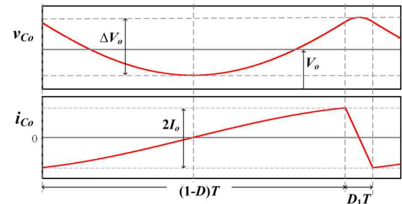
그림 13 출력필터 커패시터의 전압과 전류 파형
