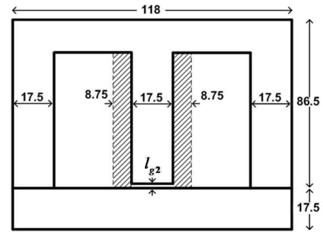
(a) 3상 코아 외형
