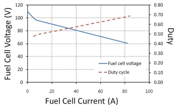
그림 15 연료전지 프로파일의 V-I 특성곡선
