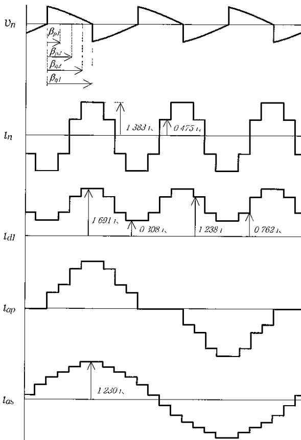
그림 6 24-펄스 시스템의 각부 파형 ( \alpha = 150^\circ )
