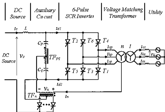
그림 1 제안하는 고펄스 SCR 인버터
