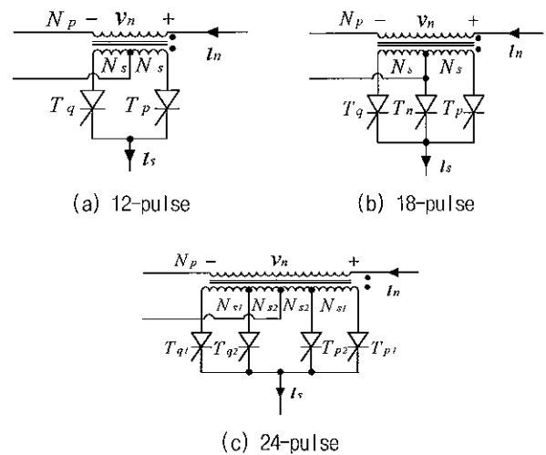
그림 2 보조싸이리스터의 연결
