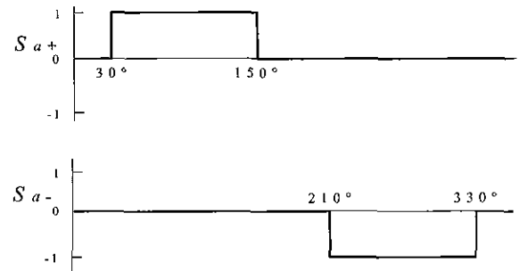
그림 5 'a' 상에 대한 스위칭 함수 S_{a+}(\alpha) 와 S_{a-}(\alpha)
