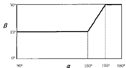
그림 3 위상각 \alpha 에 대한 최적 점화각 \beta
